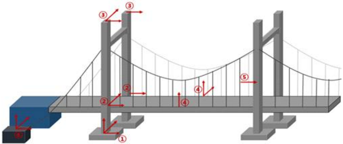
[별도 12] 현수교의 지진가속도감지기 설치 위치(제22조 관련)
